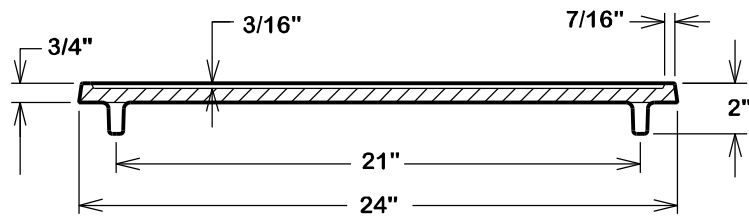
VIEW A-A
